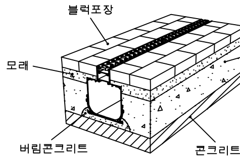
설치예시도 1 scale : None
