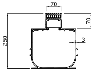
정면도 scale : None
