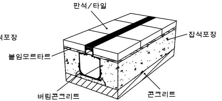
설치예시도 2 scale : None
