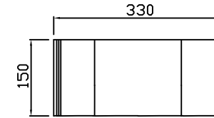
평 면 도 scale : None
