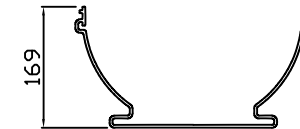
정 면 도 scale : None
