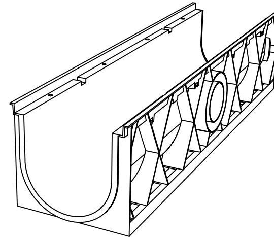
예시도 scale : None
