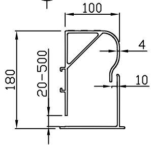
정면도 scale : None
